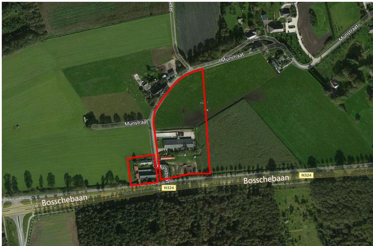
Begrenzing plangebied
