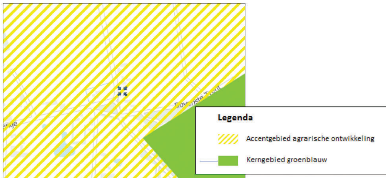
Afbeelding 4: Uitsnede structurenkaart
