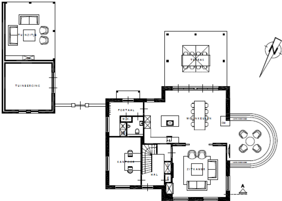
Afbeelding 16: begane grond RvR woning
