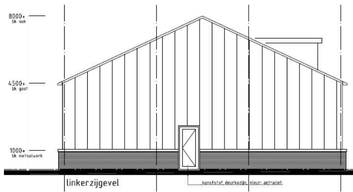
Linker zijgevel beoogde loods
