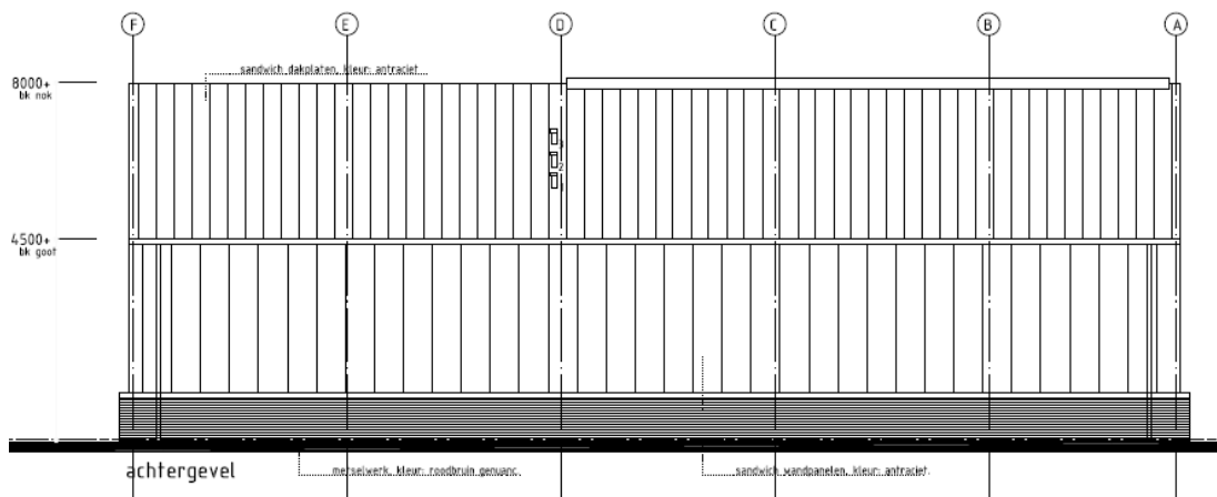
Achtergevel beoogde loods
