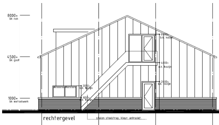
Rechter zijgevel beoogde loods
