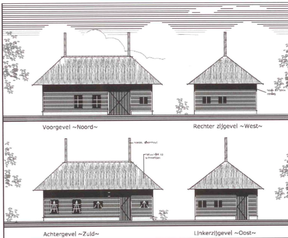
Schetsontwerp: Hooiberg Munstraat 14 te Schaijk
