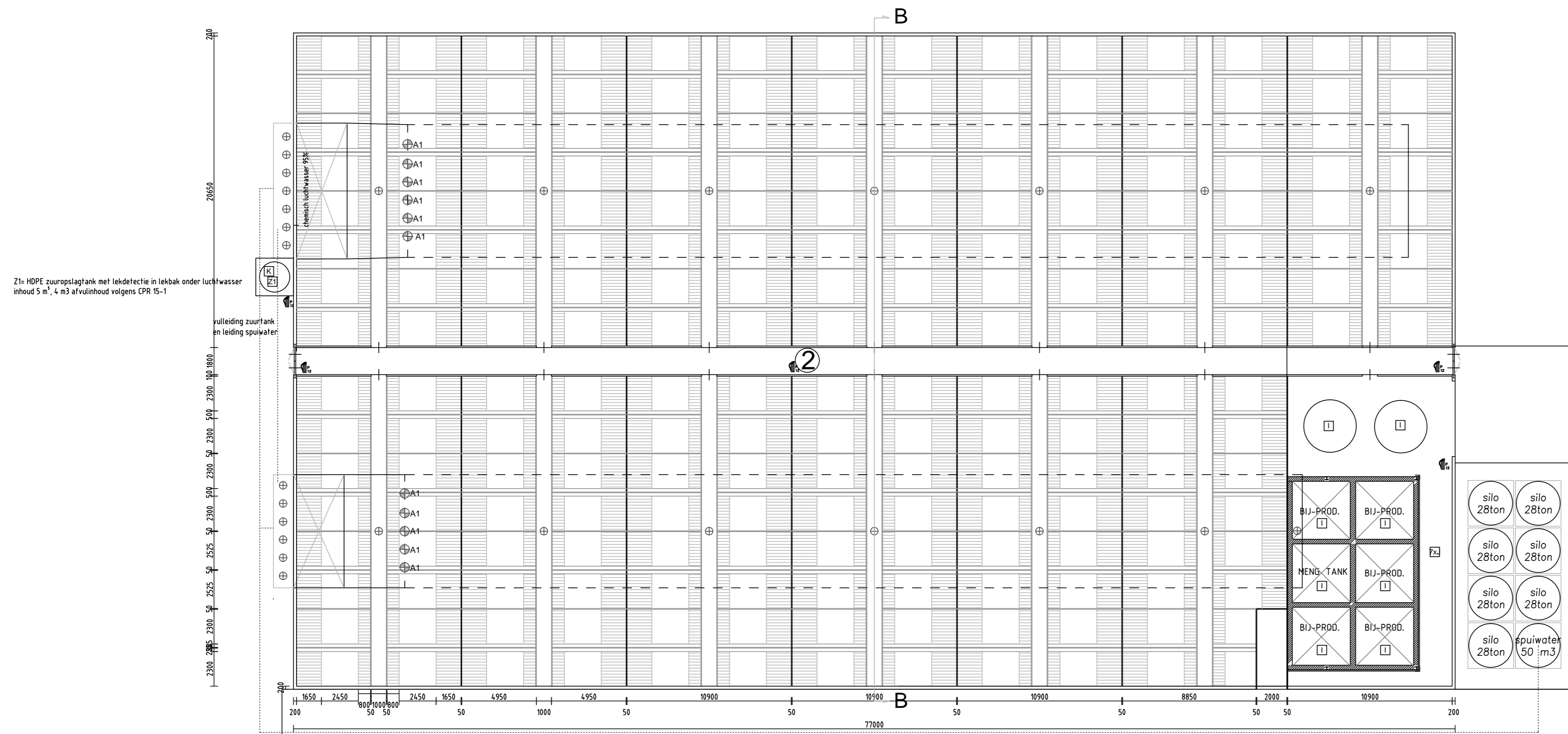
Schema chemische luchtwasser lengte wasser: per 22.500 m3 150 cm + eindstuk 60 cm
