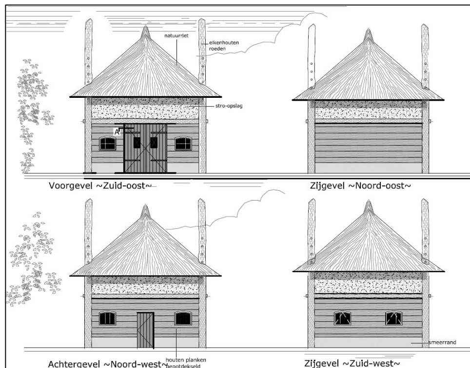
Schetsontwerp: Hooiberg Verbindingsweg 5 te Zeeland
