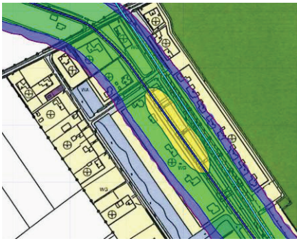
Figuur 9: PR 10^{-6} contour binnen het plangebied
