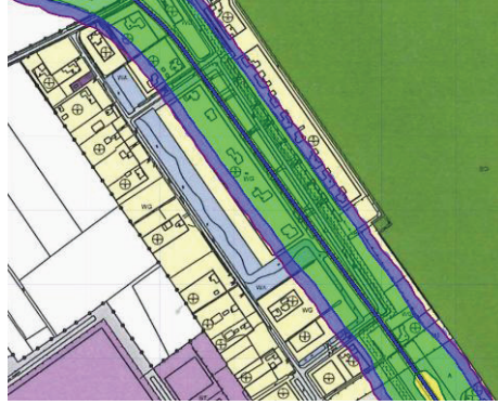
Figuur 11: Berekening na 80 cm grondoplegging
