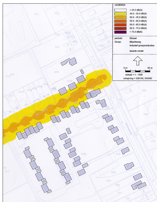
geluidscontour Mauritsweg
