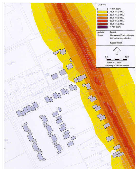
geluidscontour Nieuweweg
