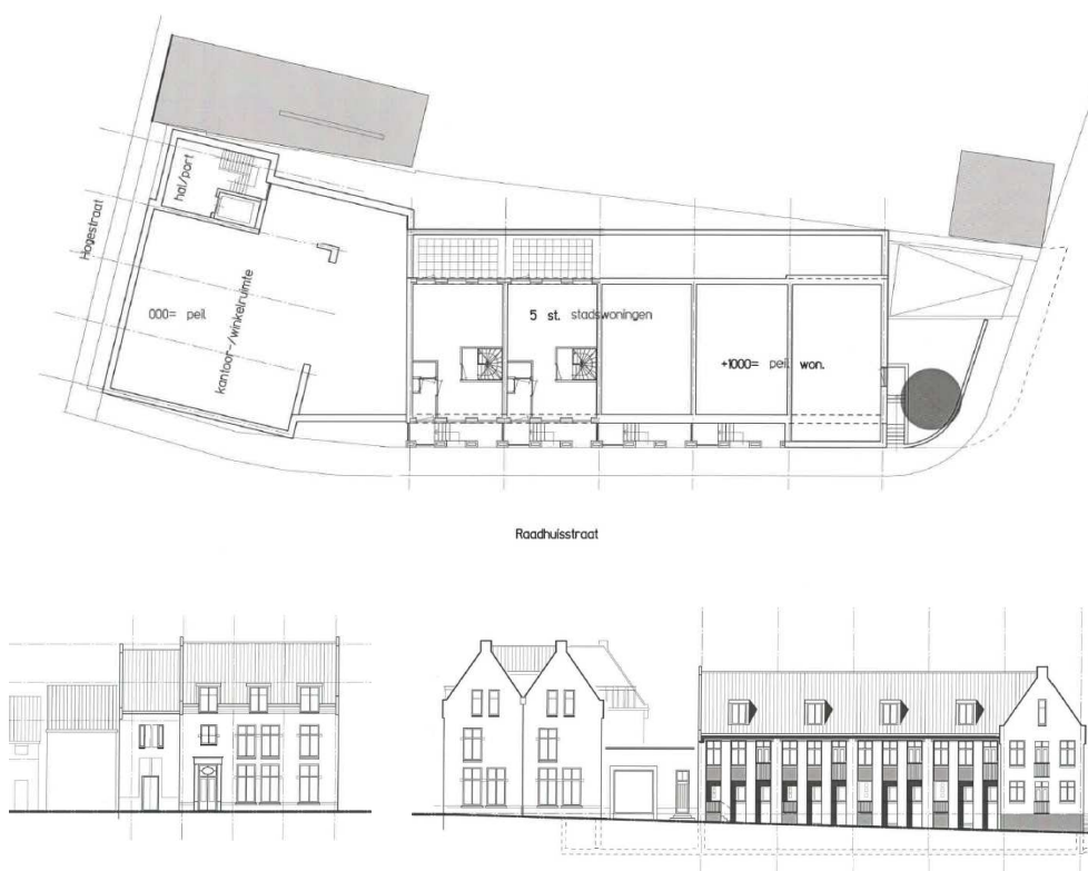
Plattegrond nieuwbouw locatie De Smid en gevelbeelden Hogestraat en Raadhuisstraat
