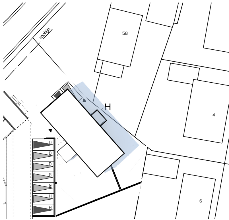
Bezonningsstudie - 21 juni 14:00 uur
