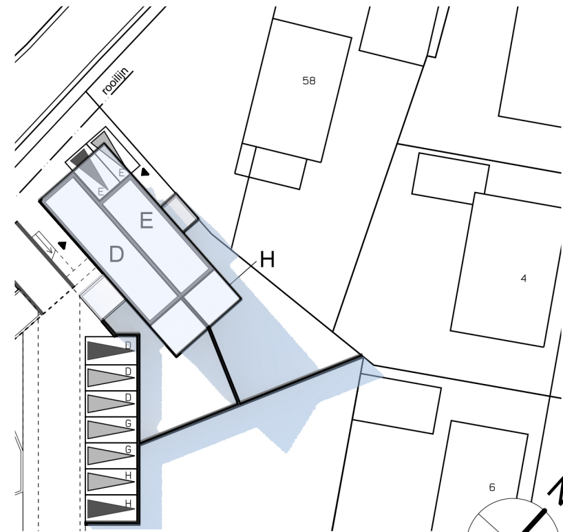
Bezonningsstudie - 21 juni 18:00 uur
