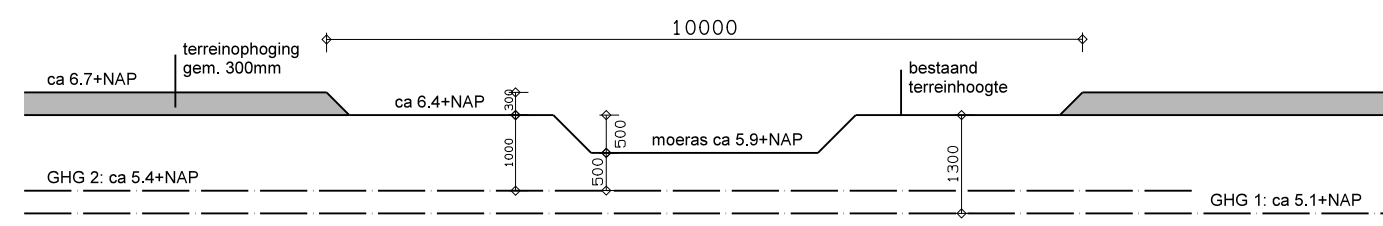
doorsnede A: moeras + infiltratie-oppervlak
