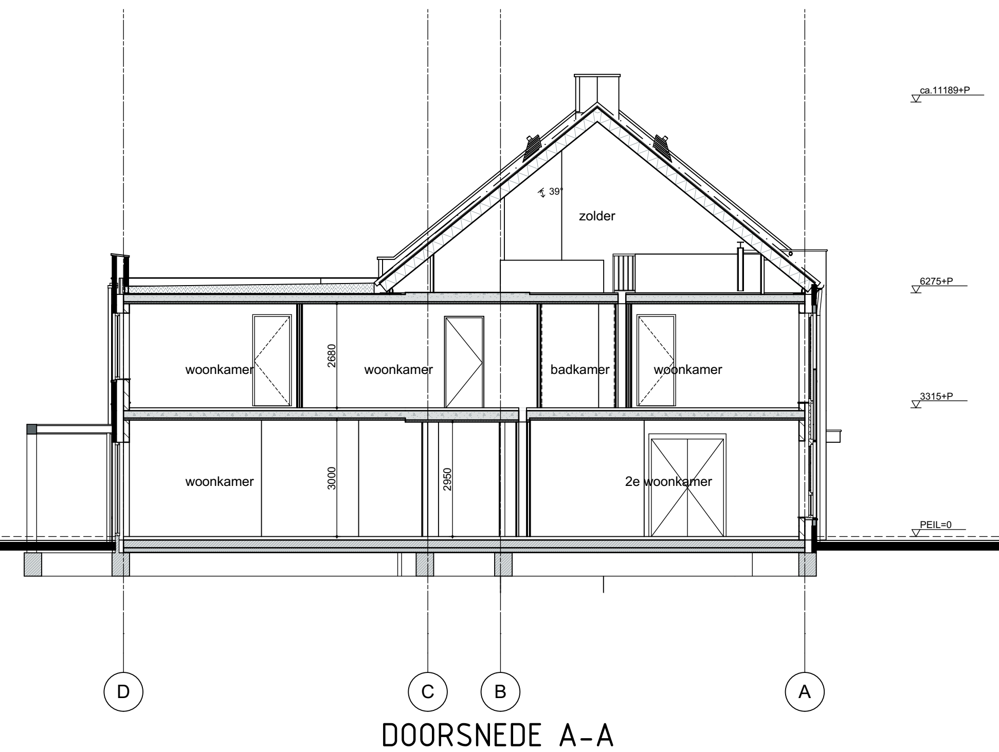
DOORSNEDE A-A
