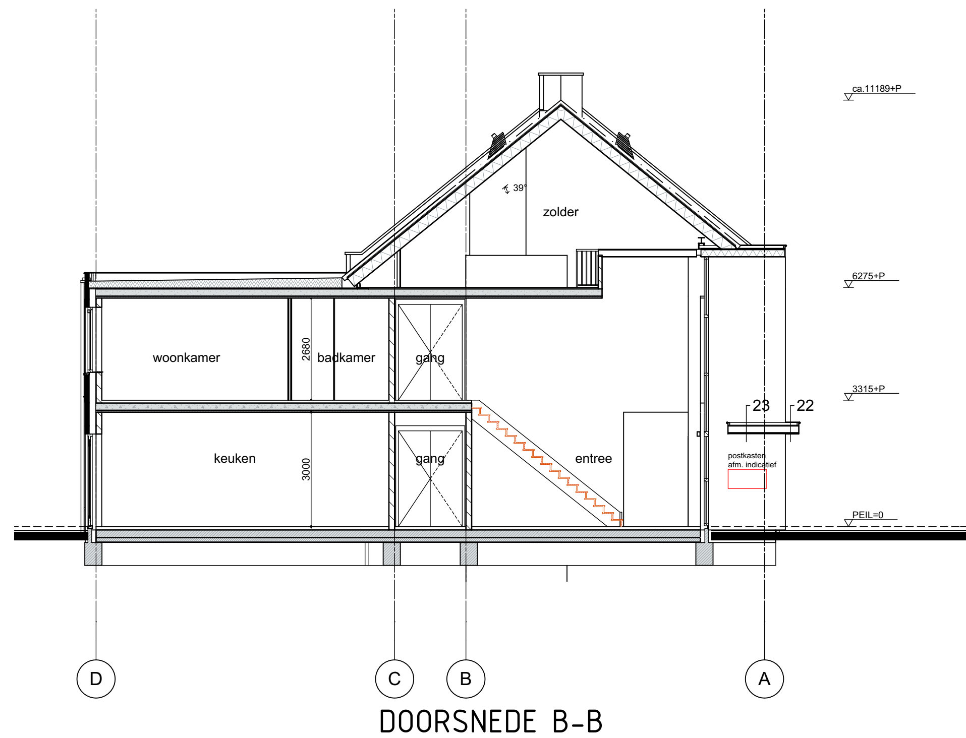
DOORSNEDE B-B
