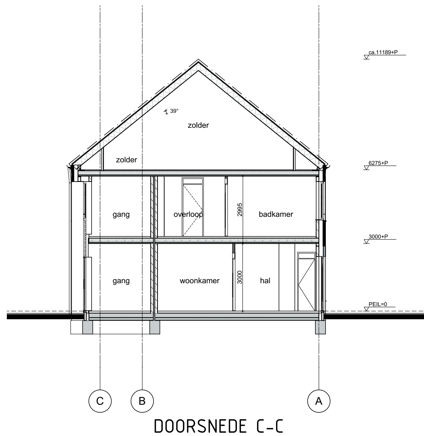
DOORSNEDE C-C
