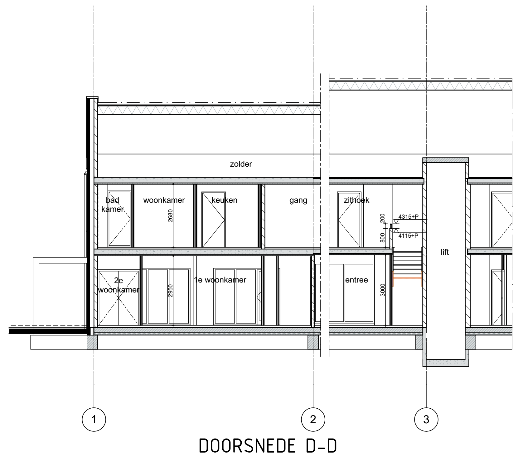
DOORSNEDE D-D
