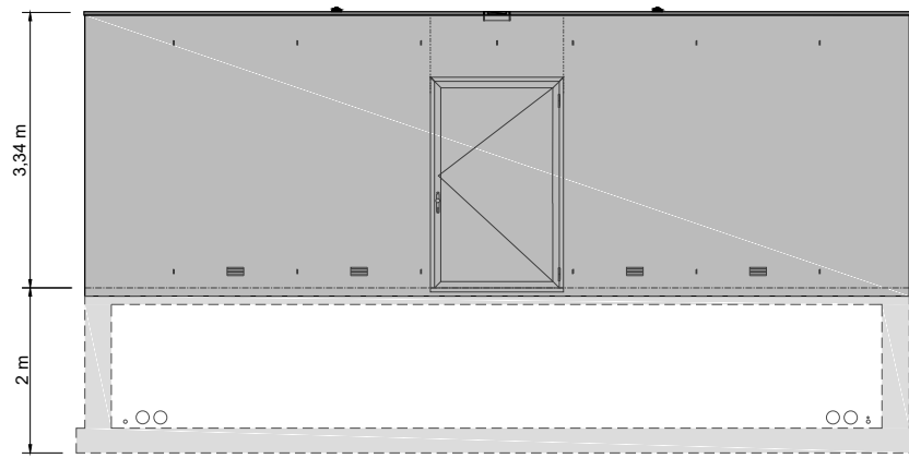
Vooraanzicht transformatorstation/ Front view transformer station
