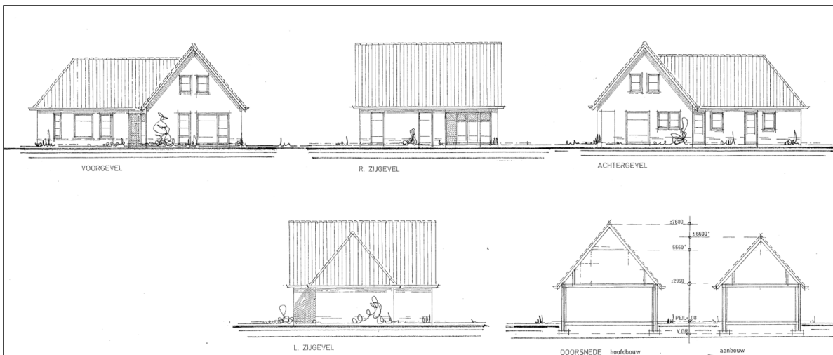
Figuur 3.3: Gevelaanzichten woning Scholtinkstraat (Bron: Morsink Architecten)
