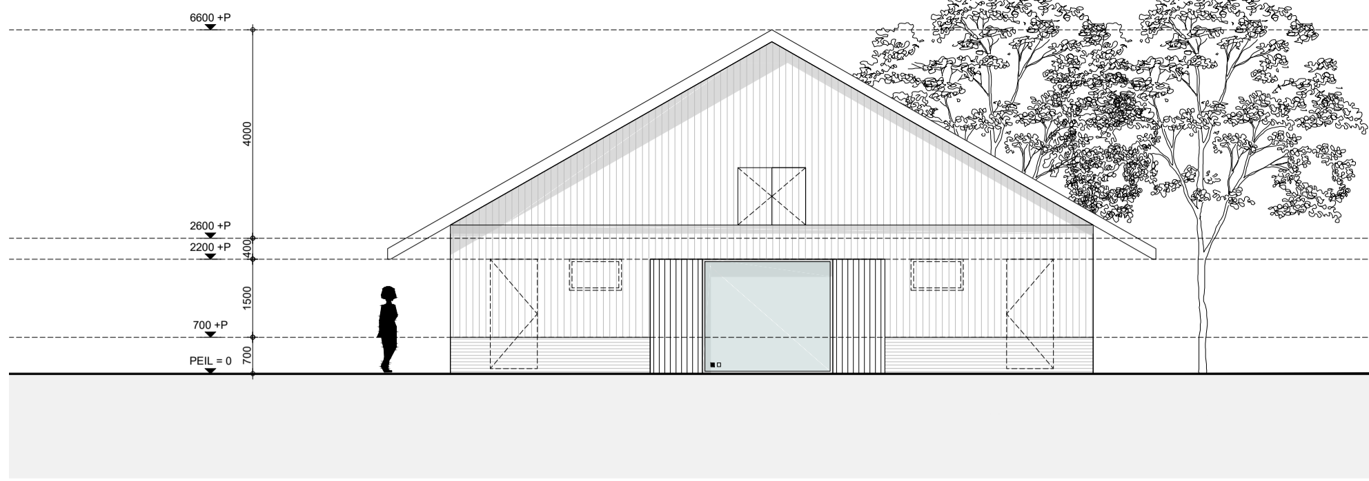
aanzicht | vooraanzicht | 1:100
