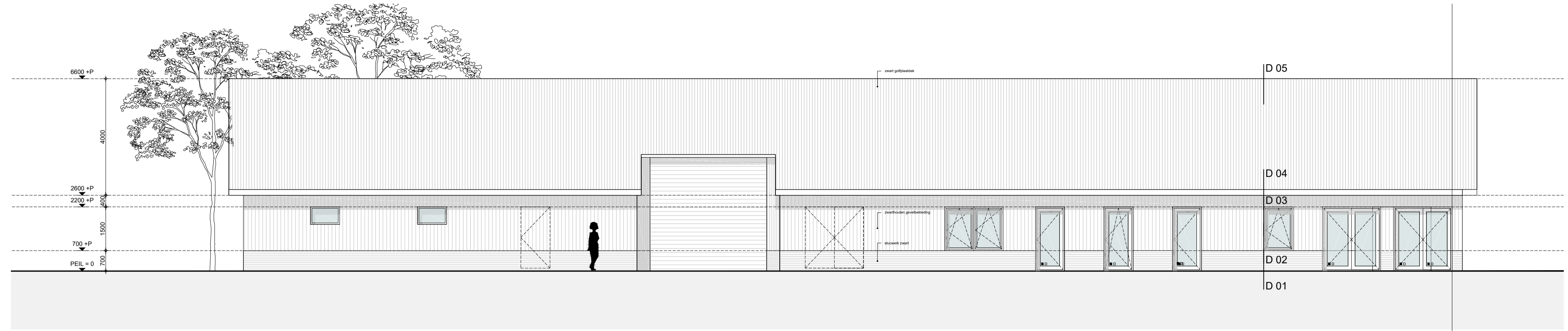
aanzicht | rechterzijanzicht | 1:100
