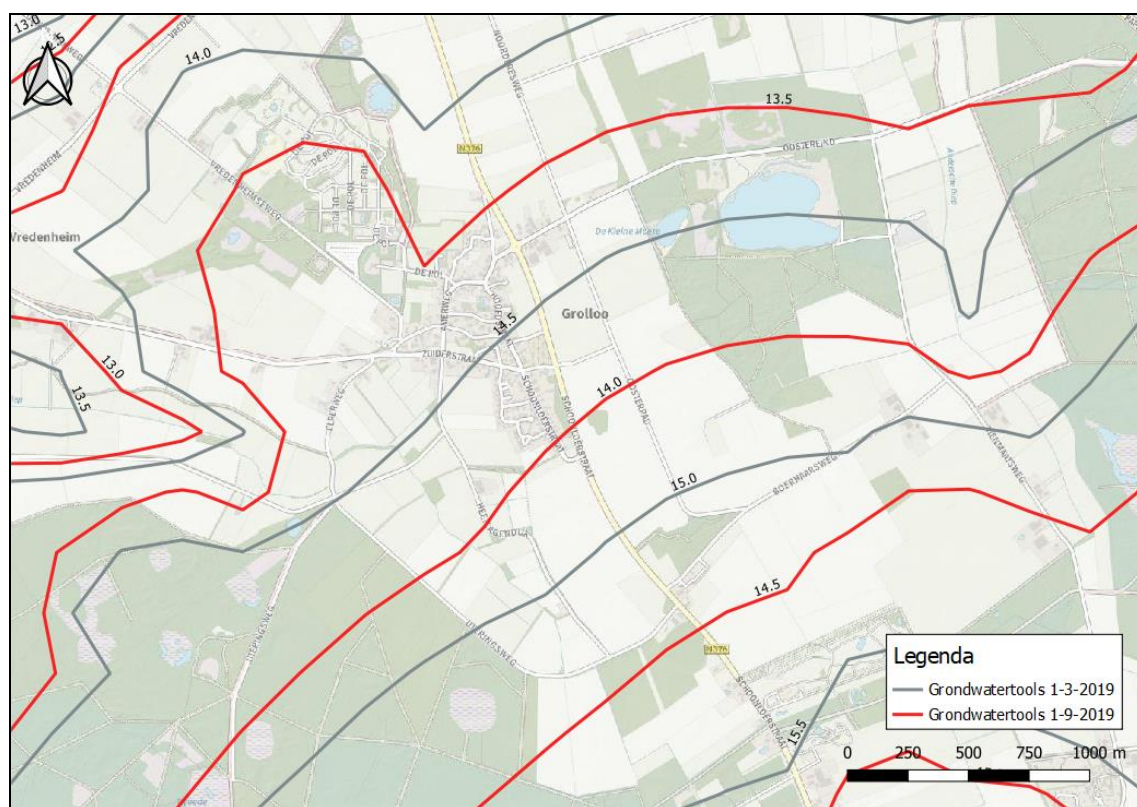
Figuur 3.3 Isohypsenvoerend pakket van stijghoogte in (bron: grondwatertools.nl)
