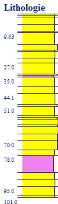
Figuur 3.1: Lokale boorprofielen TNO Dinoloket
