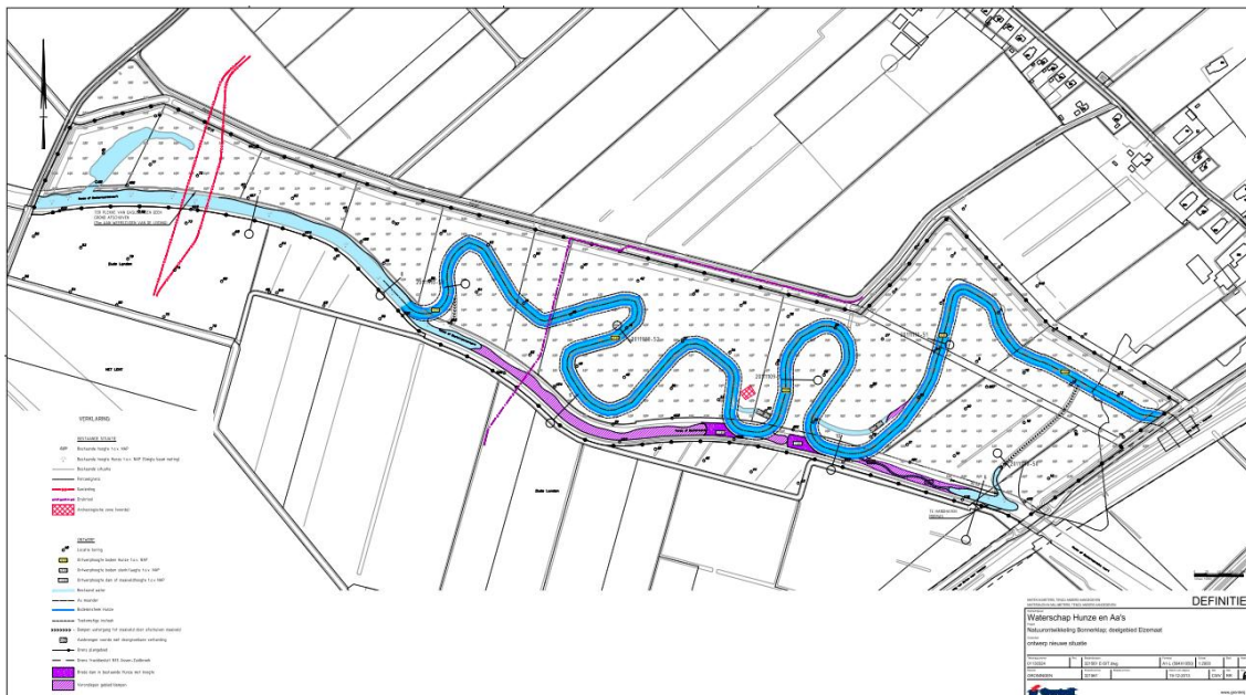
Afbeelding 4: Ontwerp verbreding meanders en dempingen
