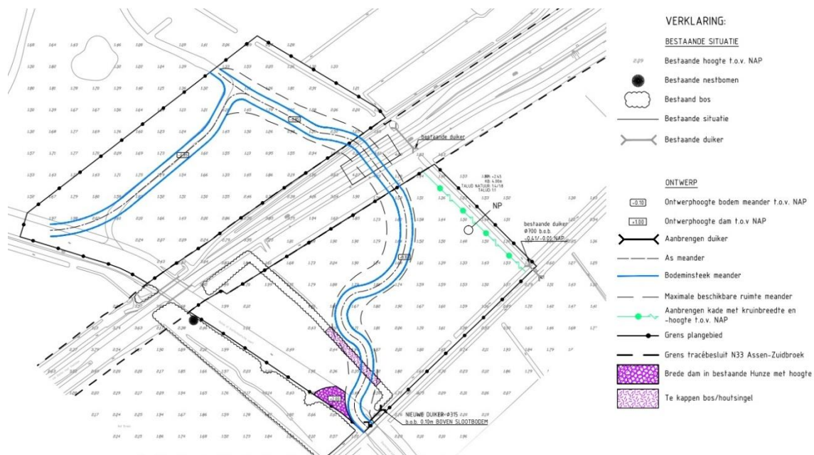
afbeelding 8: plantekening
