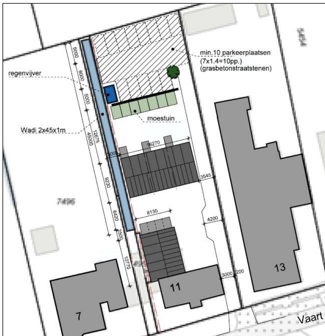
Beoogde maatregelen watercompensatie: wadi en regenvijver (bron: Tjade Timmer Architect & Bouwadvies)
