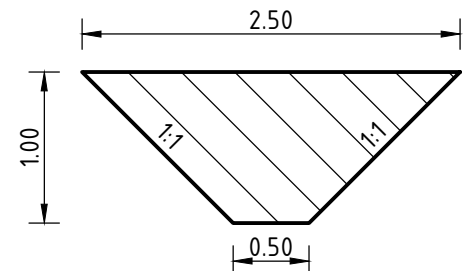
Doorsnede A-A Schaal 1:50
