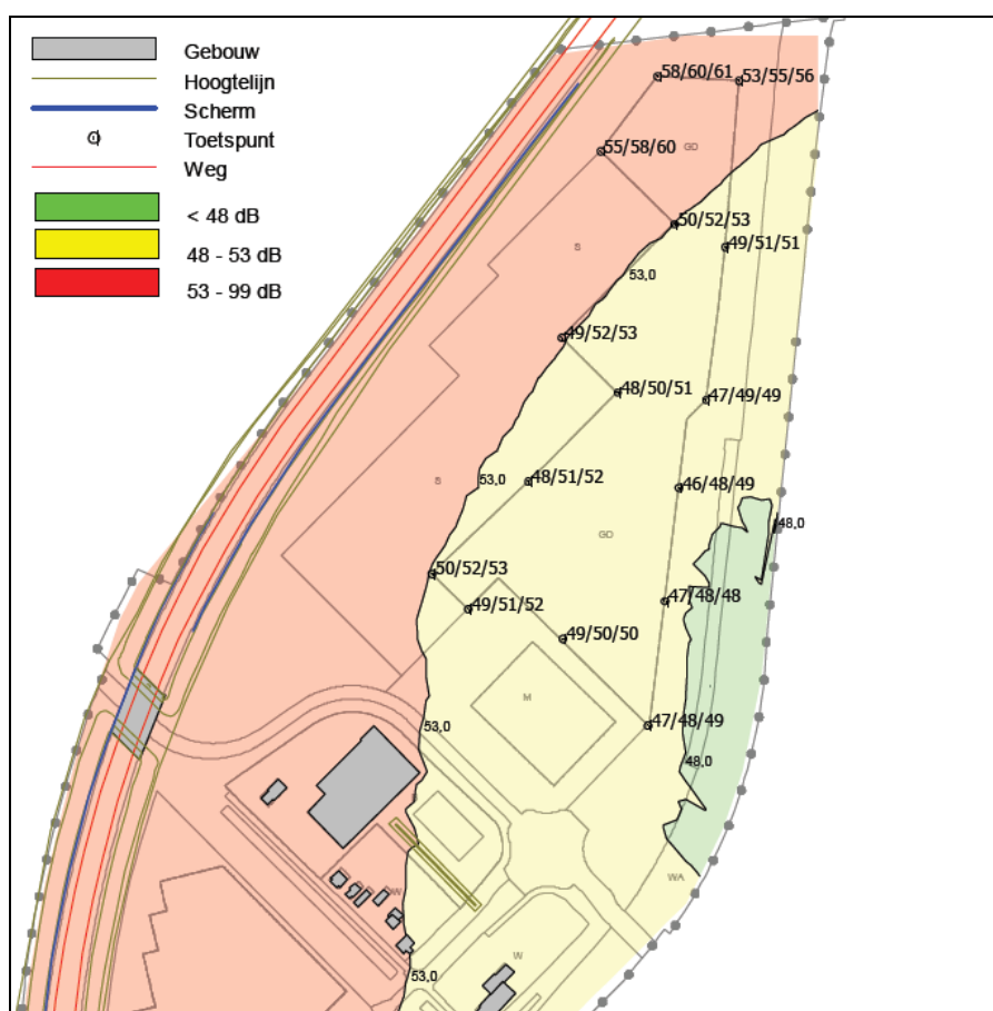
Figuur 18. Geluidsbelasting Variant 2
