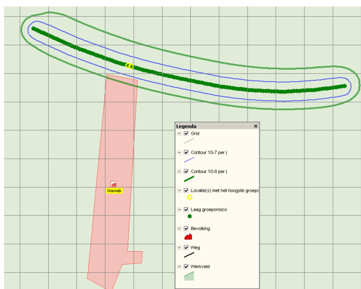
Figuur 4.3 PR10-7 en PR10-8 risicocontour in gemodelleerde omgeving van de huidige situatie
