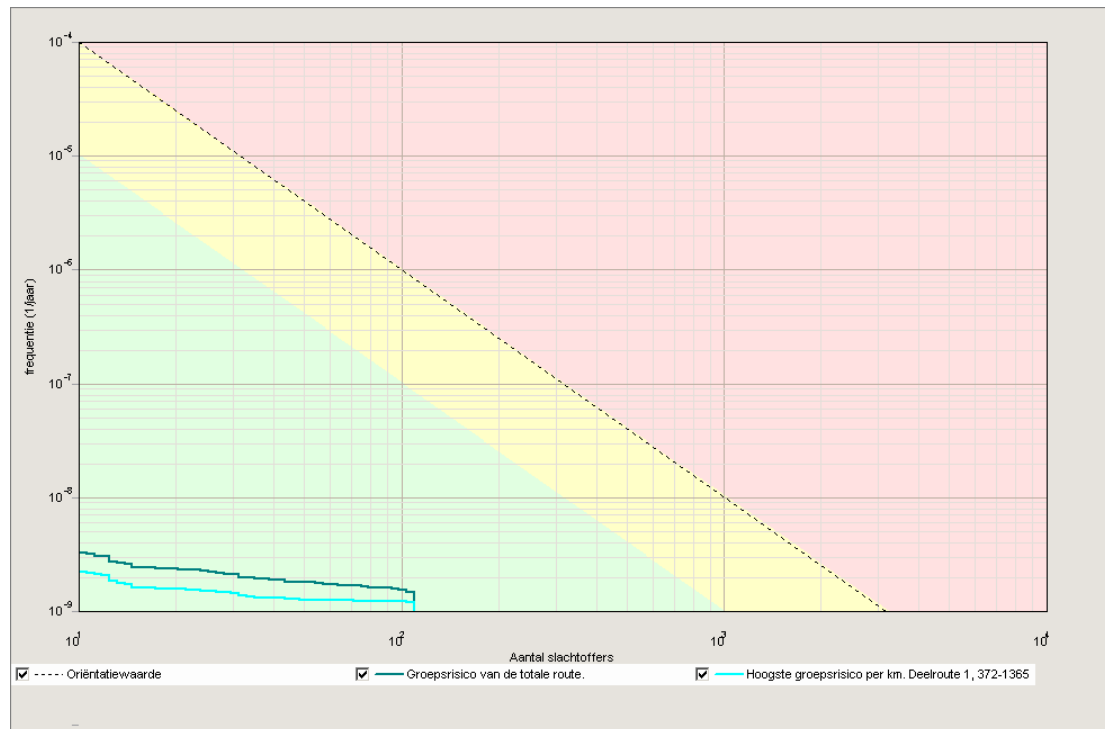
Figuur 4.5 f/N curve van het groepsrisico van de nieuwe situatie spoor
