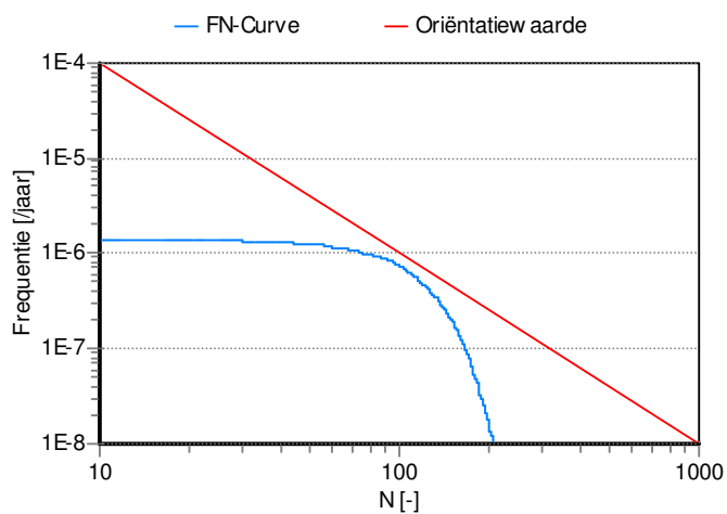
Figuur 19 FN-curve worst-casesegment 000142 met 30 cm extra dekking, nieuwe situatie. Overschrijdingsfactor 0.75.
