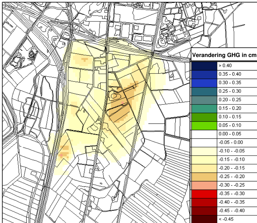
Afbeelding 33 Verandering GHG, situatie met drainage
