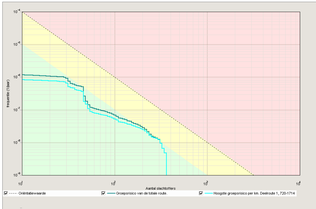
Figuur 4.3 f/N curve van het groepsrisico van de nieuwe situatie A28
