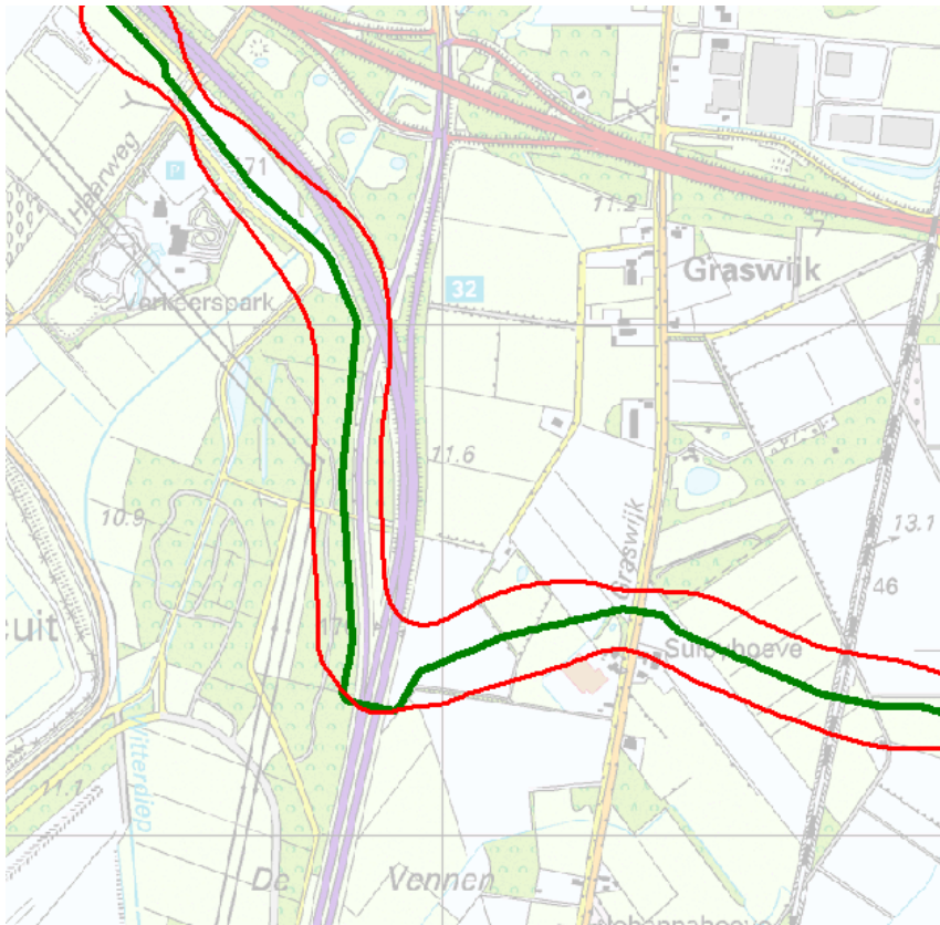
Figuur 7 Ligging van de 000142 (groen) en 10^6 per jaar PR-contouren van deze leiding (rood).
