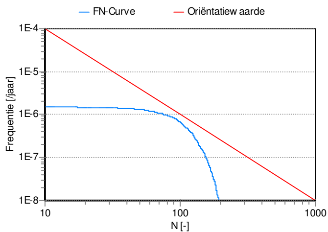
Figuur 14 FN-curve worst-casesegment 000142 bedreven op 68 bar, nieuwe situatie. Overschrijdingsfactor 0.69.
