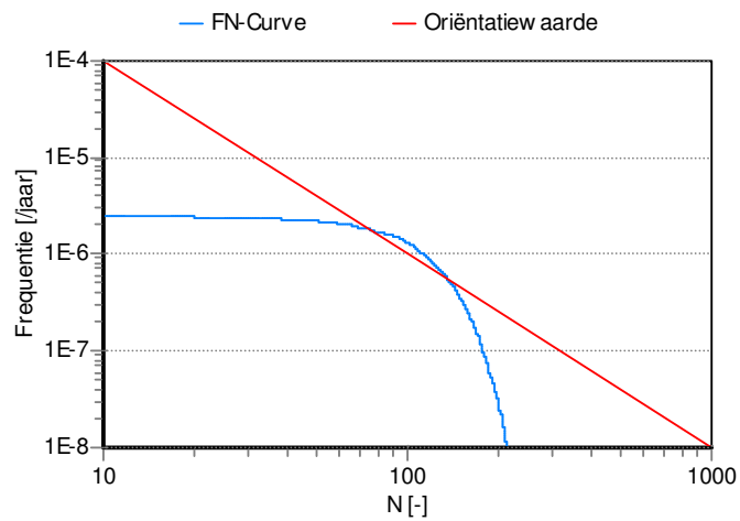
Figuur 9 FN-curve worst-casesegment 000142, nieuwe situatie. Overschrijdingsfactor 1.33.
