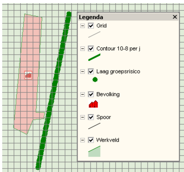
Figuur 4.5 PR10-8 risicocontour in gemodelleerde omgeving van de huidige situatie
