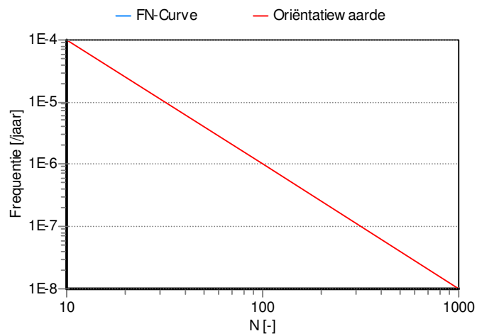
Figuur 11 FN-curve worst-casesegment 000142, bestaande situatie. Overschrijdingsfactor 0.00.
