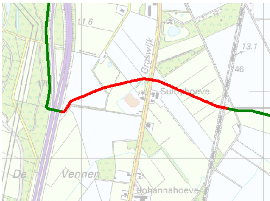
Figuur 6 Worst-casesegment van de 000132, weergegeven in rood. Dit segment levert het hoogste groepsrisico op in de nieuwe situatie.
