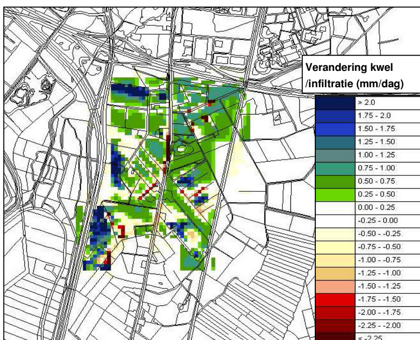
Afbeelding 34 Verandering kwel/infiltratie, wintersituatie met drainage
