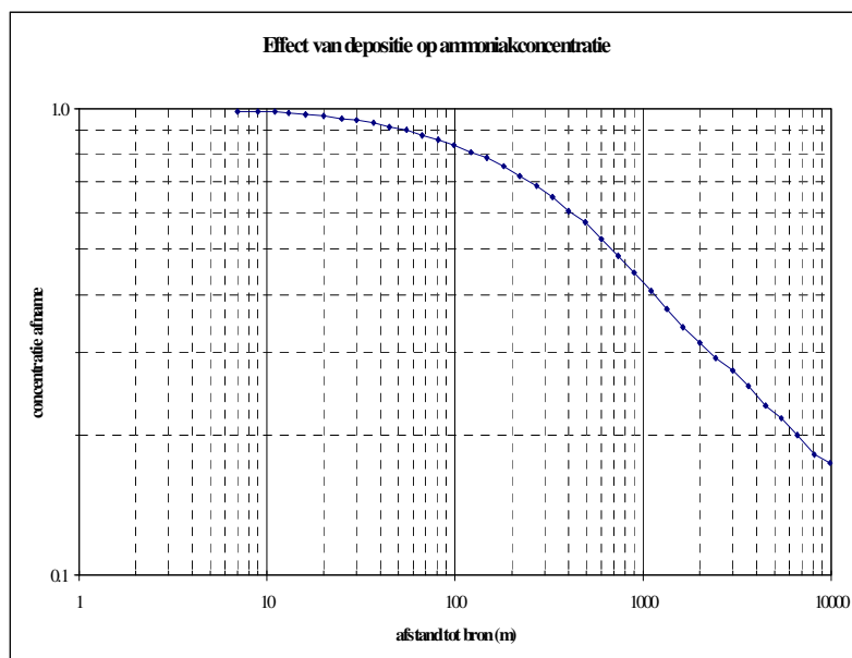
Figuur 2 Effect van depositie op de ammoniakconcentratie als functie van de afstand tot de weg (Bron: PBL, 2009).
