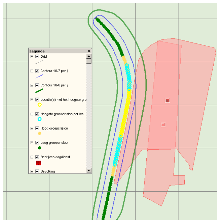
Figuur 4.2 PR10-7 en PR10-8 risicocontour in gemodelleerde omgeving van de nieuwe situatie met plan
