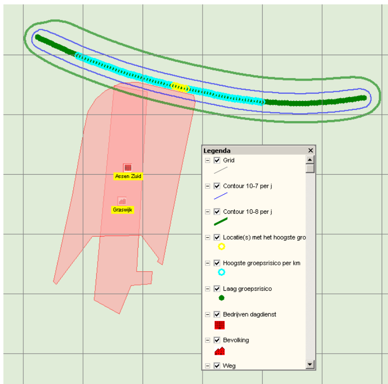
Figuur 4.4 PR10-7 en PR10-8 risicocontour in gemodelleerde omgeving van de nieuwe situatie met plan
