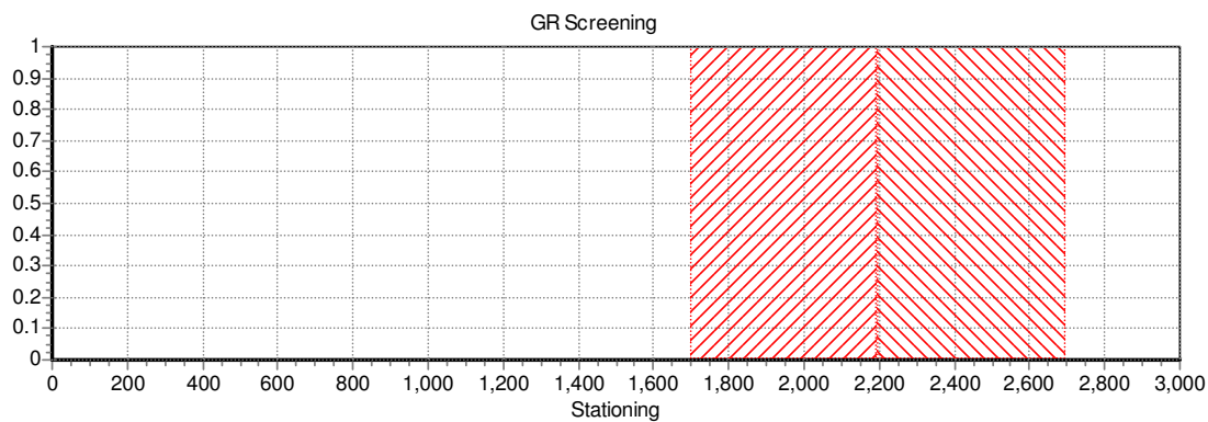
Figuur 20 Overschrijdingsfactor uitgezet tegen stationing van de 000142 met 30 cm extra dekking, bestaande situatie. Het rood gearceerd deel geeft de kilometer aan waarover de FN-curve is berekend.
