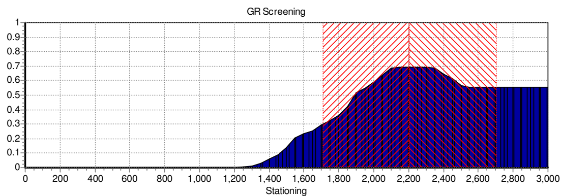
Figuur 13 Overschrijdingsfactor uitgezet tegen stationing van de 000142 bedreven op 68 bar, nieuwe situatie. Het rood gearceerde deel geeft de kilometer aan waarover de FN-curve is berekend.
