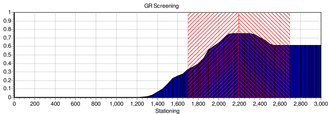
Figuur 18 Overschrijdingsfactor uitgezet tegen stationing van de 000142 met 30 cm extra dekking, nieuwe situatie. Het rood gearceerde deel geeft de kilometer aan waarover de FN-curve is berekend.
