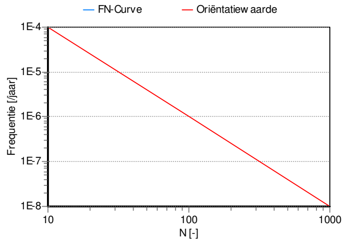
Figuur 21 FN-curve worst-casesegment 000142 met 30 cm extra dekking, bestaande situatie. Overschrijdingsfactor 0.00.
