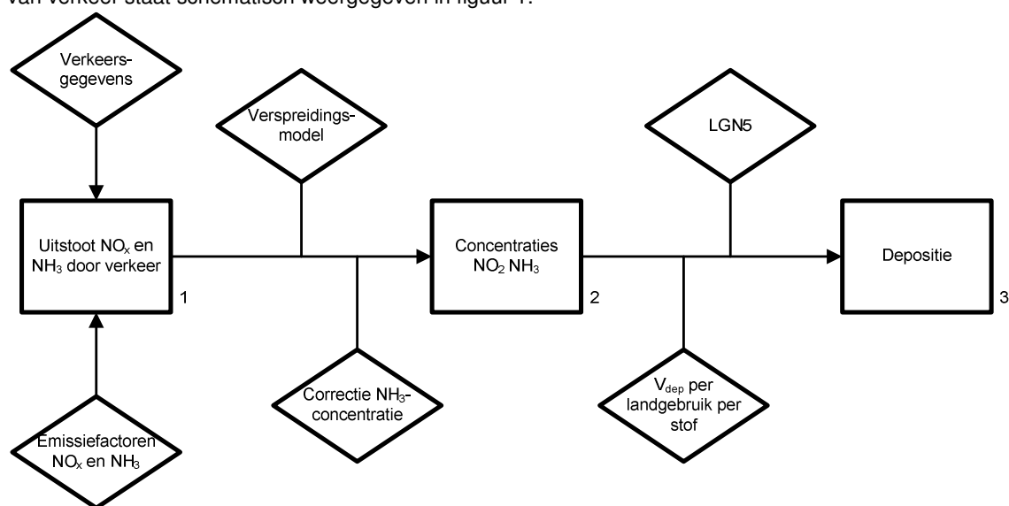
Figuur 1 Schematische weergave van de methodiek ter bepaling stikstofdepositie als gevolg van verkeer.
