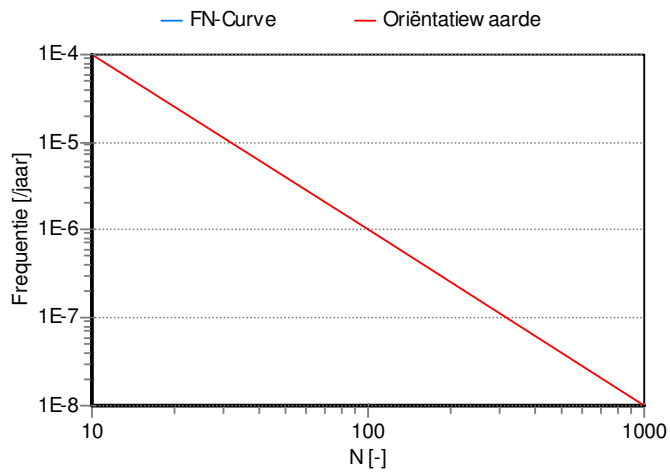
Figuur 5 FN-curve worst-casesegment 000132, bestaande situatie. Overschrijdingsfactor 0.00.
