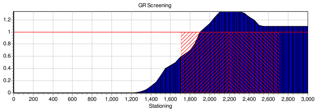
Figuur 8 Overschrijdingsfactor uitgezet tegen stationing van de 000142, nieuwe situatie. Het rood gearceerde deel geeft de kilometer aan waarover de FN-curve is berekend.
