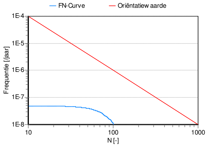
Figuur 3 FN-curve worst-casesegment 000132, nieuwe situatie. Overschrijdingsfactor 0.01.
