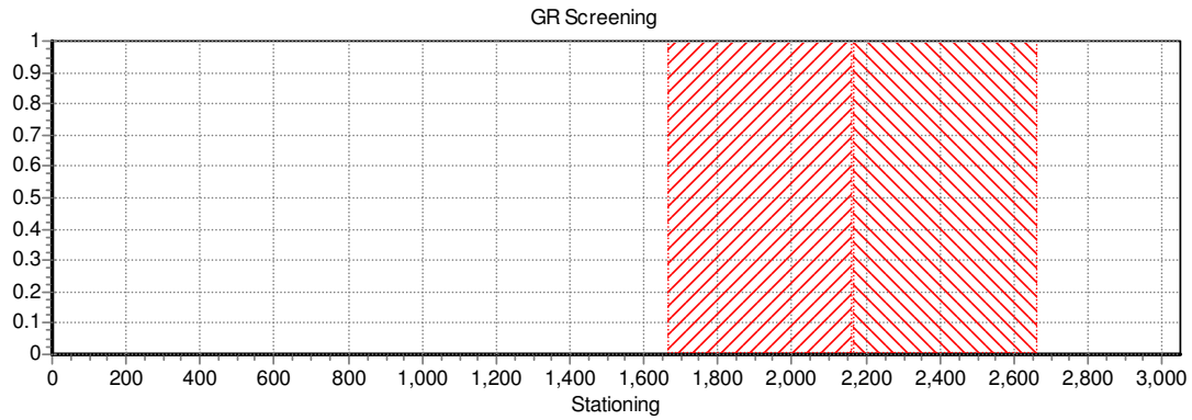
Figuur 4 Overschrijdingsfactor uitgezet tegen stationing van de 000132, bestaande situatie. Het rood gearceerde deel geeft de kilometer aan waarover de FN-curve is berekend.
