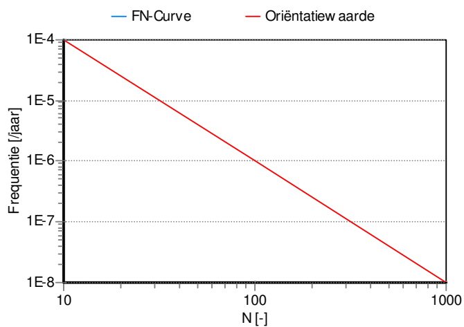
Figuur 16 FN-curve worst-casesegment 000142 bedreven op 68 bar, bestaande situatie. Overschrijdingsfactor 0.00.
