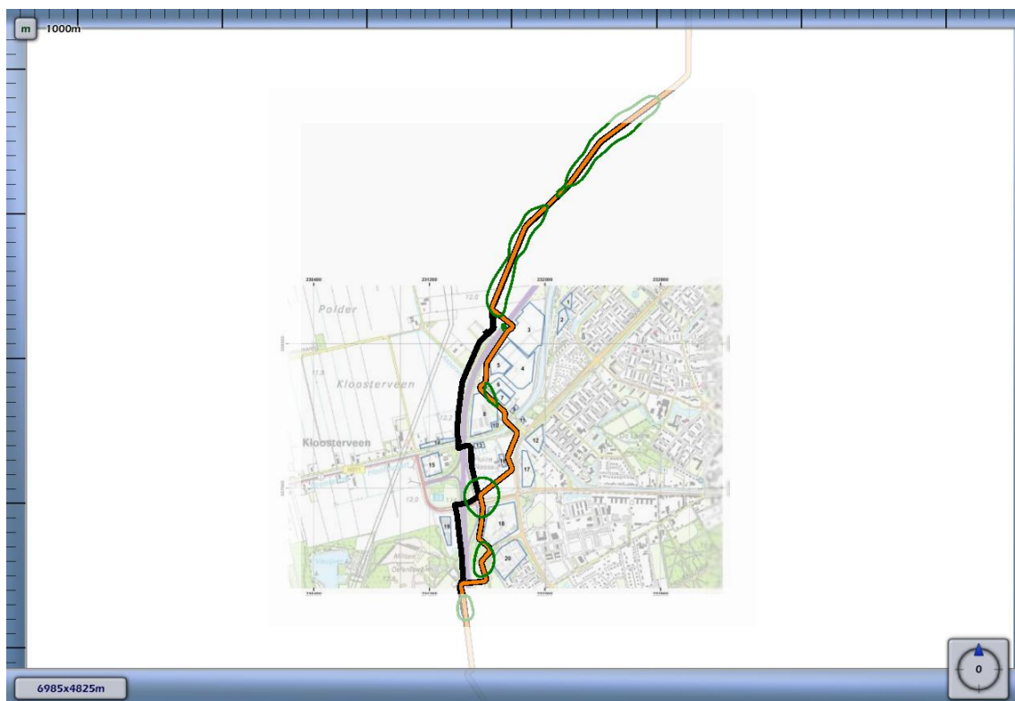
3.1 Figuur 3.1 Plaatsgebonden risico voor {95652112-6439-472F-8831-17463BAAB3DB}_000132 van NAM BV
