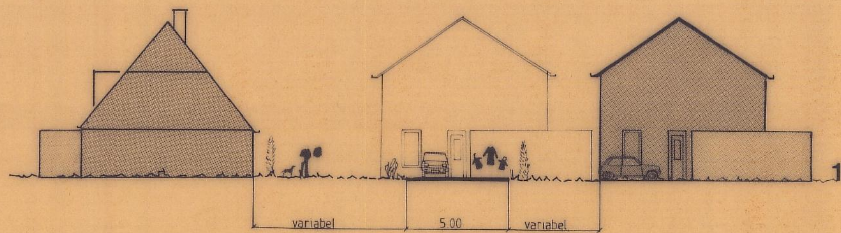
DWARSPROFIEL SCHAAL 1:200
