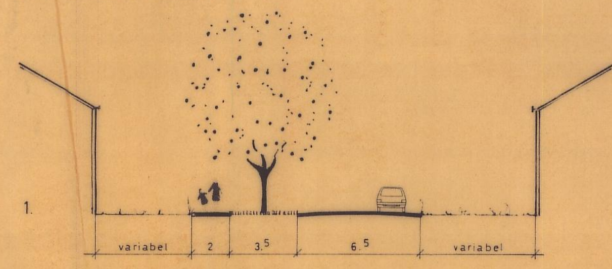
DWARSPROFIEL SCHAAL 1:200
