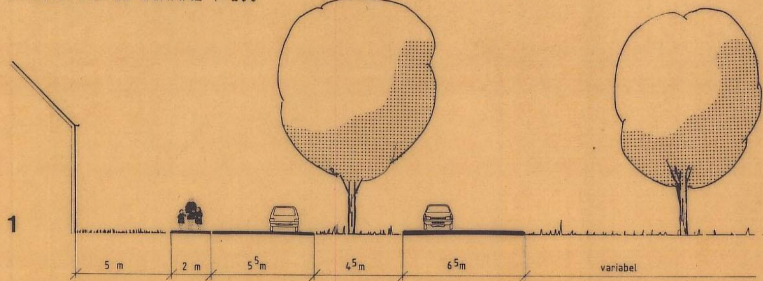
DWARSPROFIEL SCHAAL 1:200
