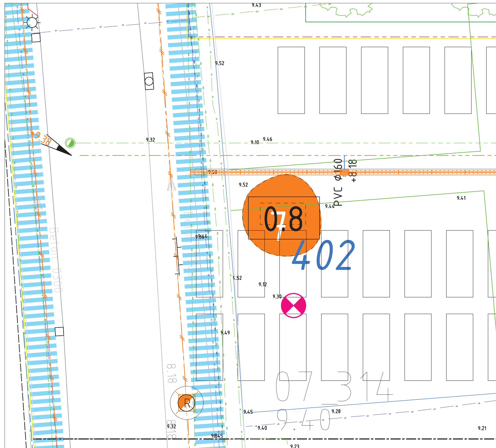
Figuur B5.6 Ontgravingscontour werkzaamheden binnen saneringslocatie 7
