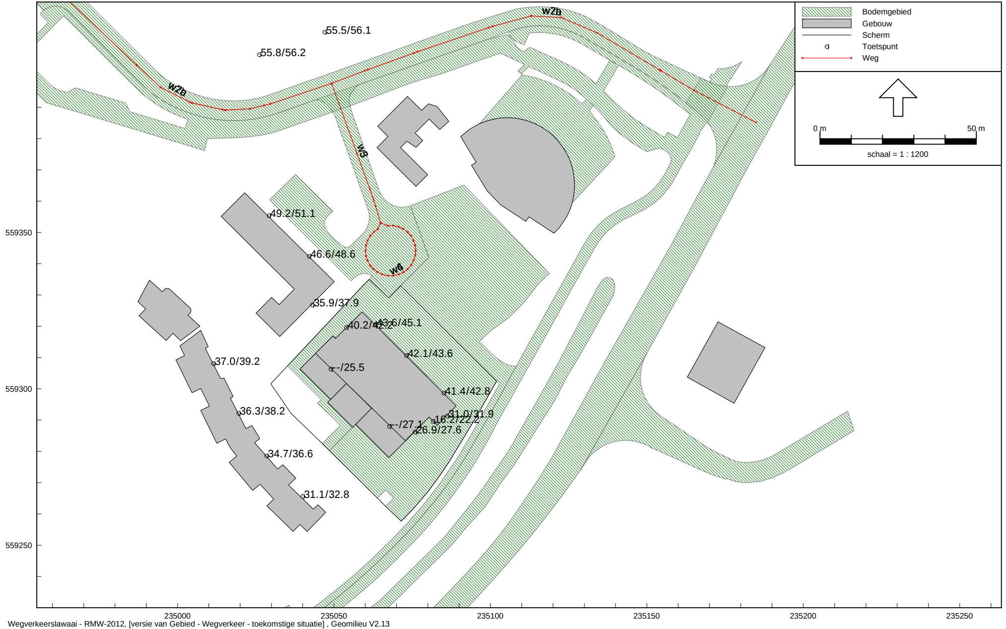
Overzicht van het rekenmodel met de berekende geluidsbelasting vanwege de M.L. Kingweg Toekomstige situatie - incl. correctie o.g.v. art. 110g
