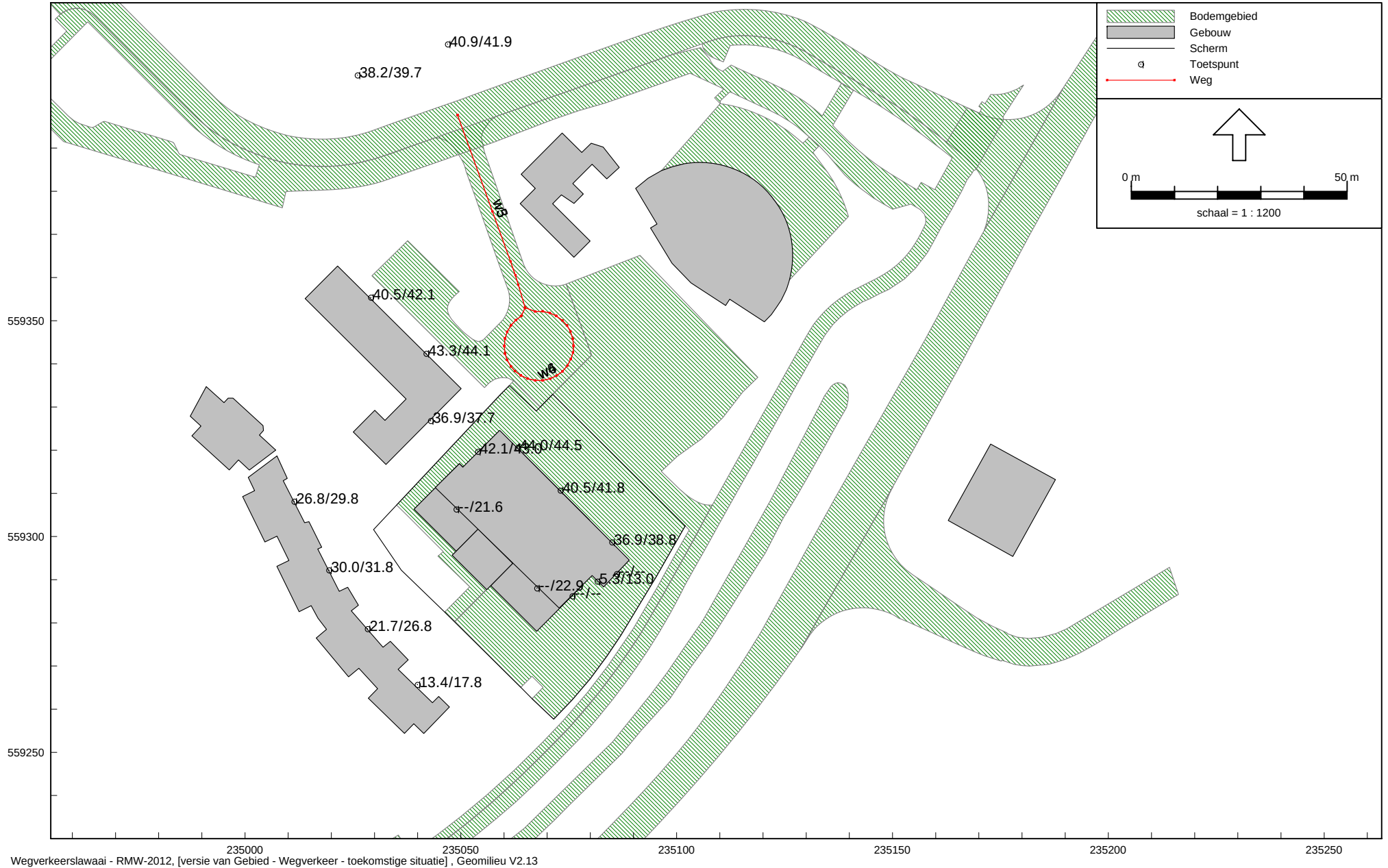
Overzicht van het rekenmodel met de berekende geluidsbelasting verkeer op de toegangsweg indirecte hinder - toekomstige situatie (dagperiode)
