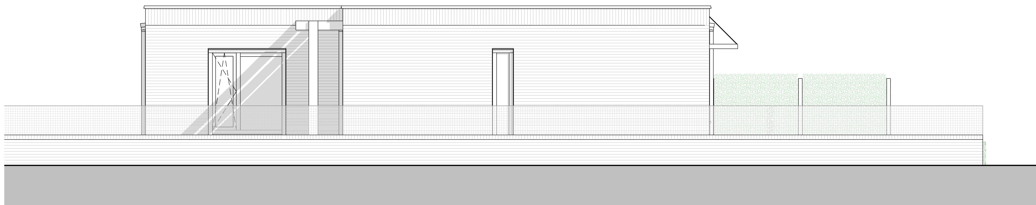
zijgevel bnr18
