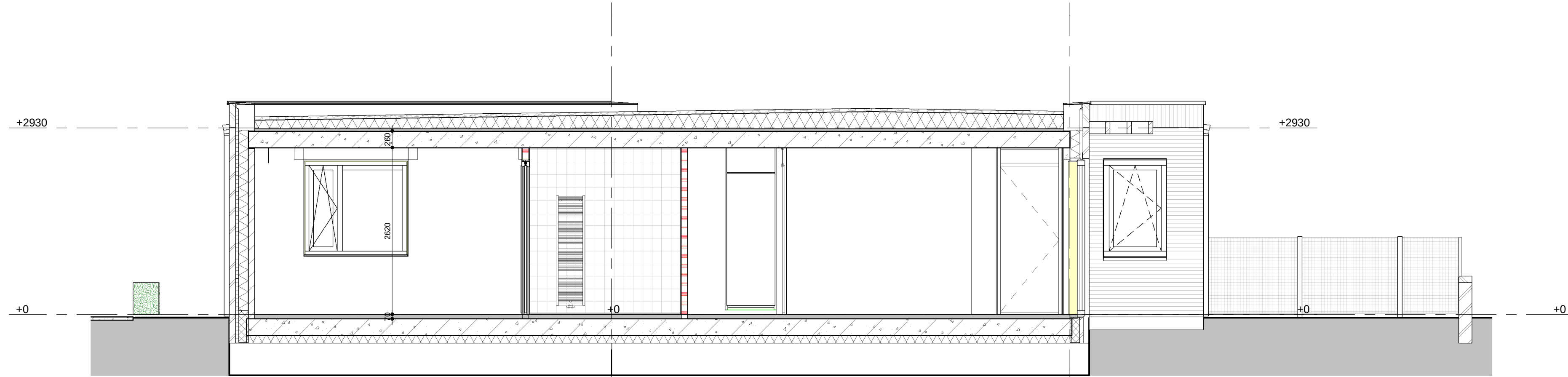
doorsnede 1-1
