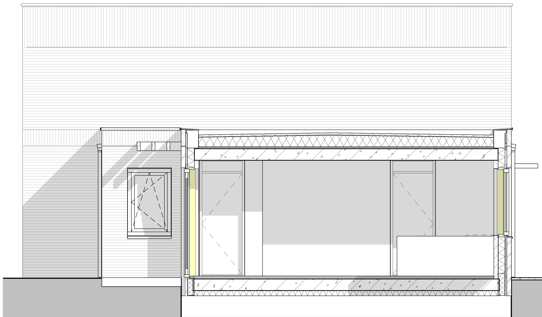
zijgevel bnr 11
