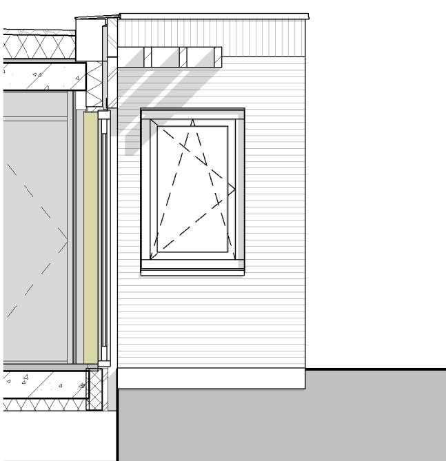
zijgevel achterzijde bnr15
