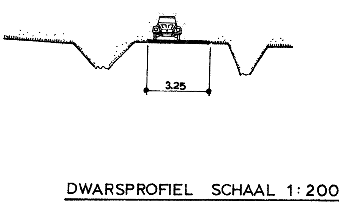
DWARSPROFIEL SCHAAL 1:200
