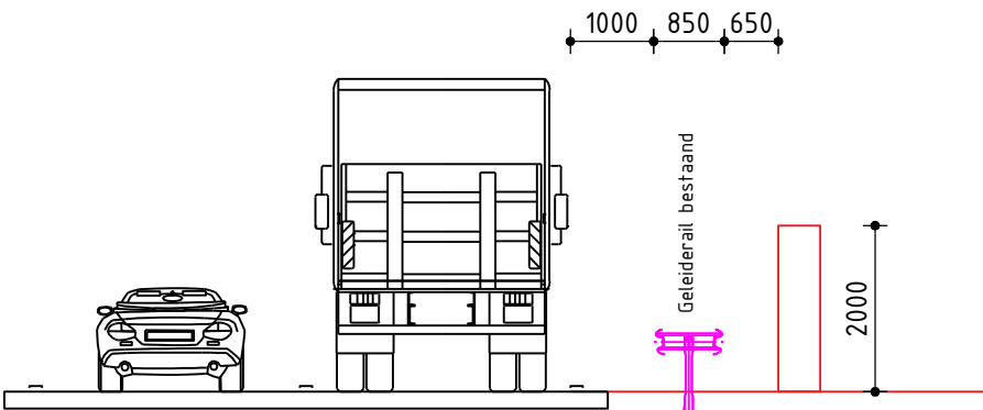
Profiel geluidsscherm Schaal 1:100
