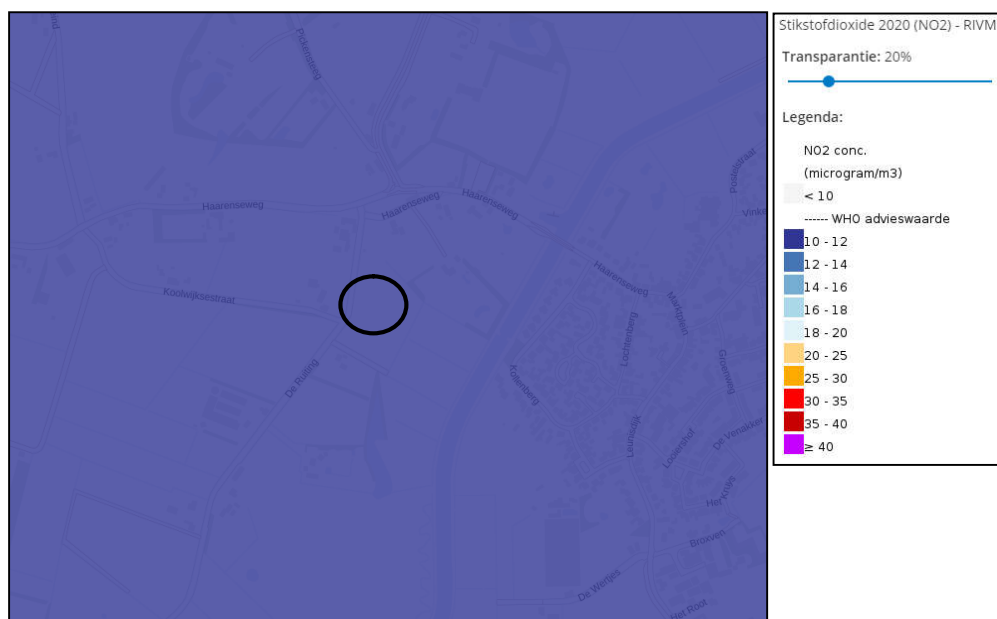
Figuur 33: Stikstofdioxide NO 2 2019 (Bron: Atlas leefomgeving)
