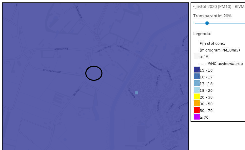
Figuur 31: Fijn stof PM 10 2020 (Bron: Atlas Leefomgeving)
