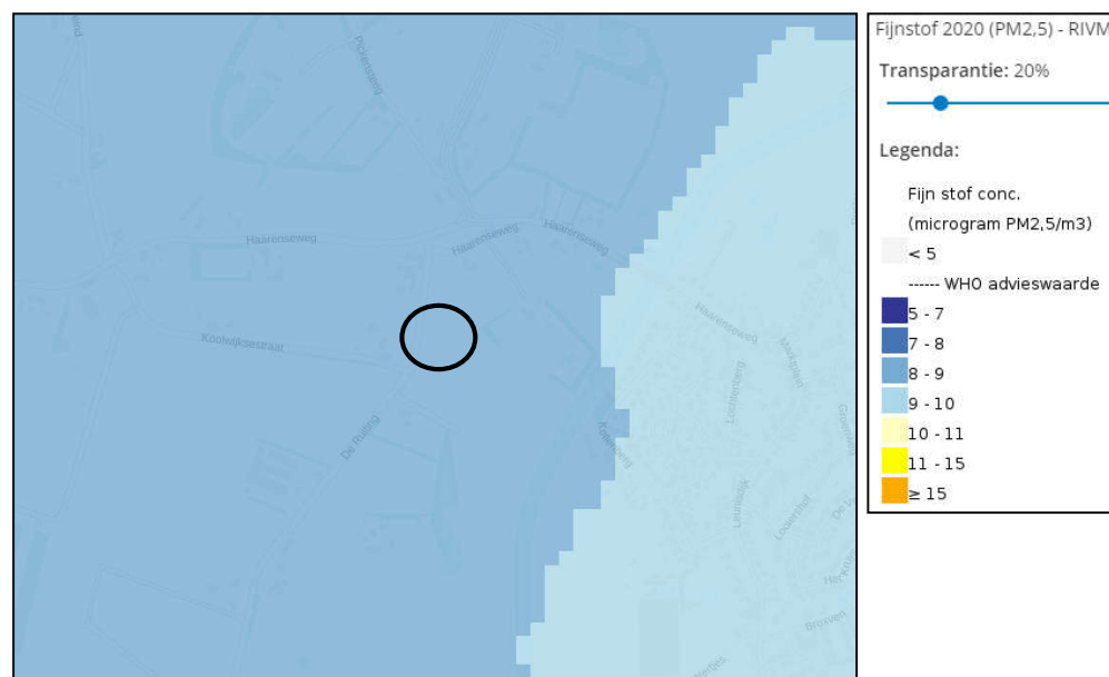
Figuur 32: Fijn stof PM 2,5 2020 (Bron: Atlas Leefomgeving)
