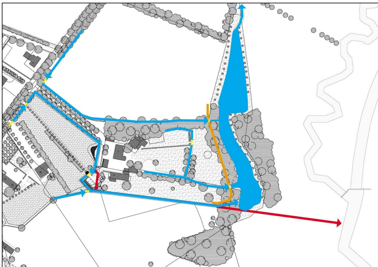
Figuur 20: Aanpassing van de detailafwatering van De Roudonck met in rood de te dempen B-wateren. In oranje is de nieuwe steilrand langs de oude visplas aangegeven. Het oppervlaktewater is weergegeven in blauwe met in geel de kunstwerken (duikers en klepduikers). De sloten centraal op de locatie -de oude omgrachting- betreft C-wateren
