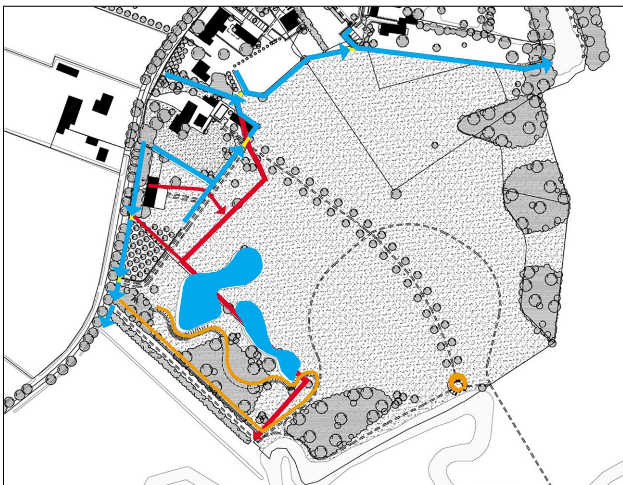
Figuur 35: Aanpassing van de detailafwatering van Landgoed De Ruiting met in rood de te dempen B- en C-wateren. De te dempen diepe sloot kent straks geen functie meer. De andere sloten worden gedempt in het kader van de terreinaanpassing. De diepe afwateringssloot die het water richting een pomp voert is een B-water, de gebogen greppel tussen twee weilanden is een C-water. Alle oppervlaktewater is weergegeven in blauw met in geel de kunstwerken (duikers). Ook hier ontbreekt een deel
