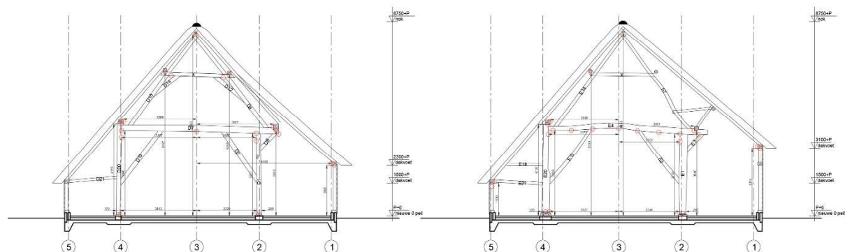
DWARSDOORSNEDE D-D
