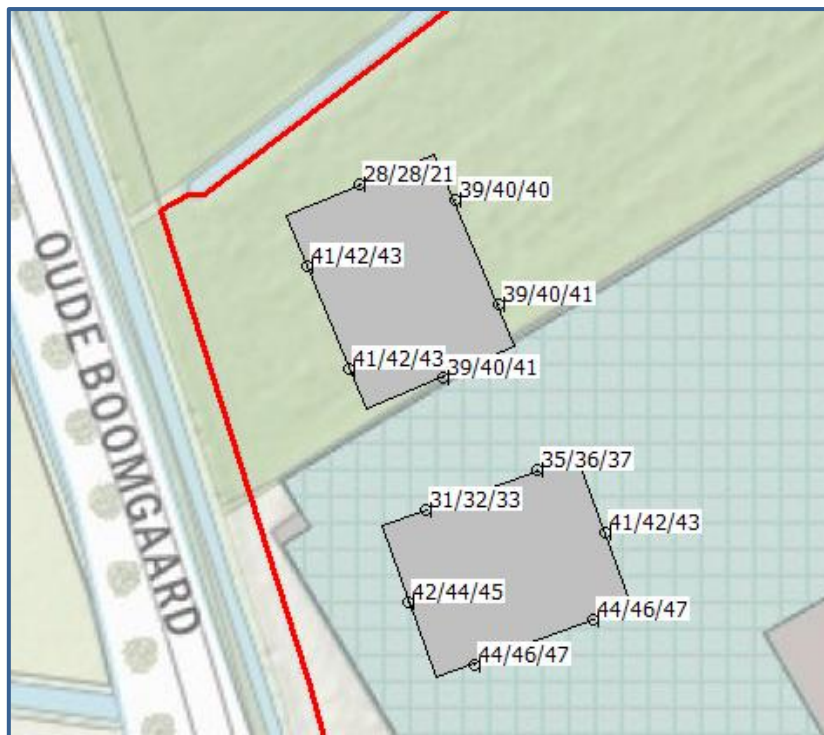
Afbeelding 7. Geluidbelastingen L den (incl. aftrek art. 110g Wgh) Schijndelsedijk Berekende geluidbelastingen op een hoogte van 1,5 / 4,5 / 7,5 meter
