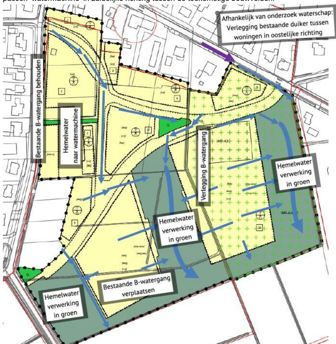
Figuur 4.3: Globale verwerkingswijze hemelwater
