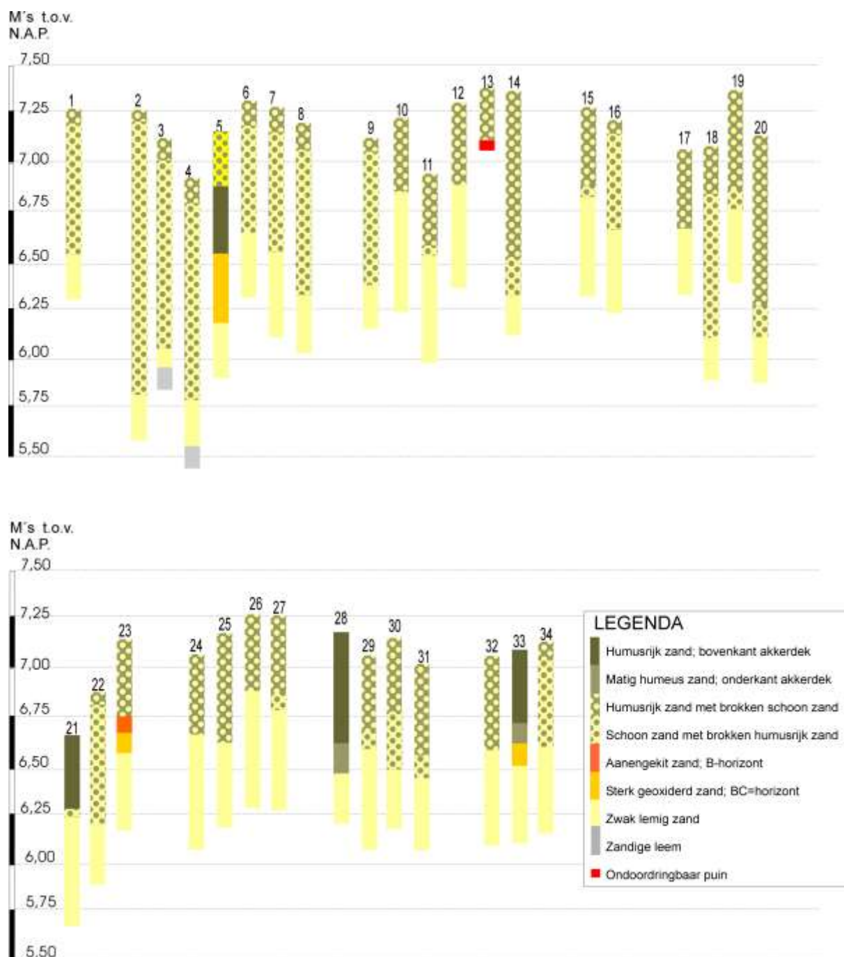
Figuur 9: Boorprofielen
