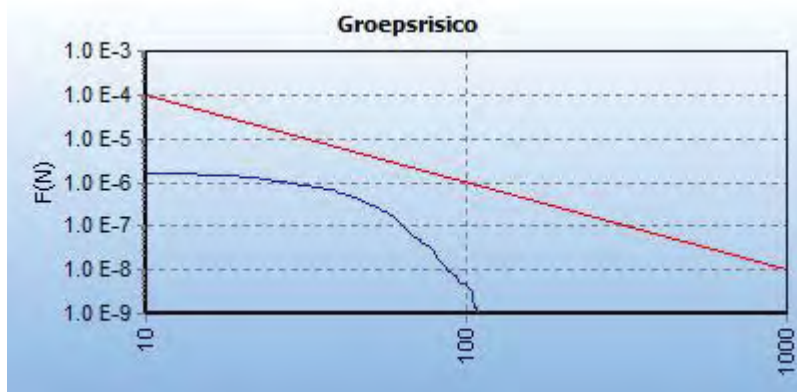
Figuur 3.2b: Groepsrisico hogedruk aardgastransportleiding Z-544-01 (toekomstige situatie)
