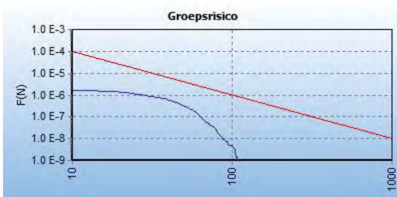
Figuur B1.4b: Groepsrisico hogedruk aardgastransportleiding Z-544-01 in de toekomstige situatie
