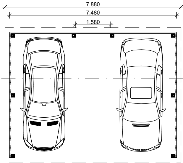
plattegrond
