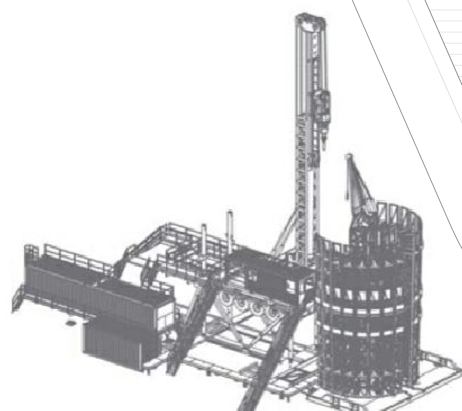
ZIJAANZICHT BOORTOREN OOSTZIJDE
