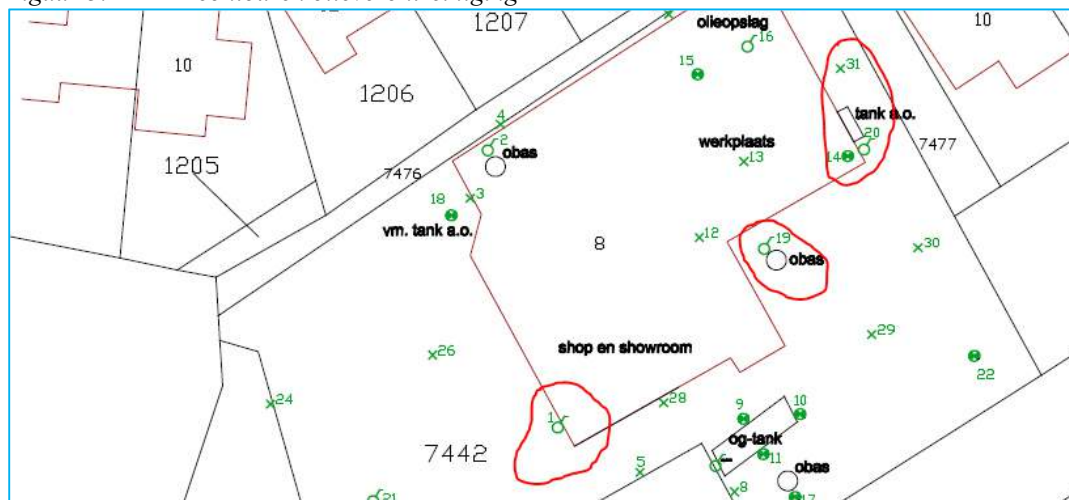
Figuur 3: contouren olieverontreiniging
