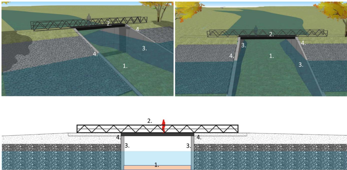
Figuur 1. Functionele onderdelen instroomvoorziening
