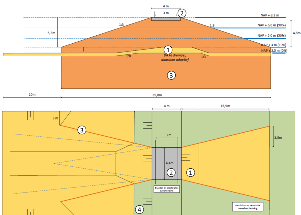
Figuur 4.: Impressie van de uitstroomvoorziening met daarin aangegeven de verschillende functionele onderdelen. Boven een dwarsdoorsnede, onder een bovenaanzicht.
