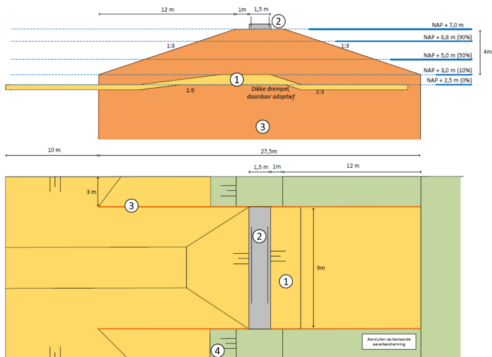
Figuur 2. Impressie van de instroomvoorziening met daarin aangegeven de verschillende functionele onderdelen. Boven een dwarsdoorsnede, onder een bovenaanzicht.
