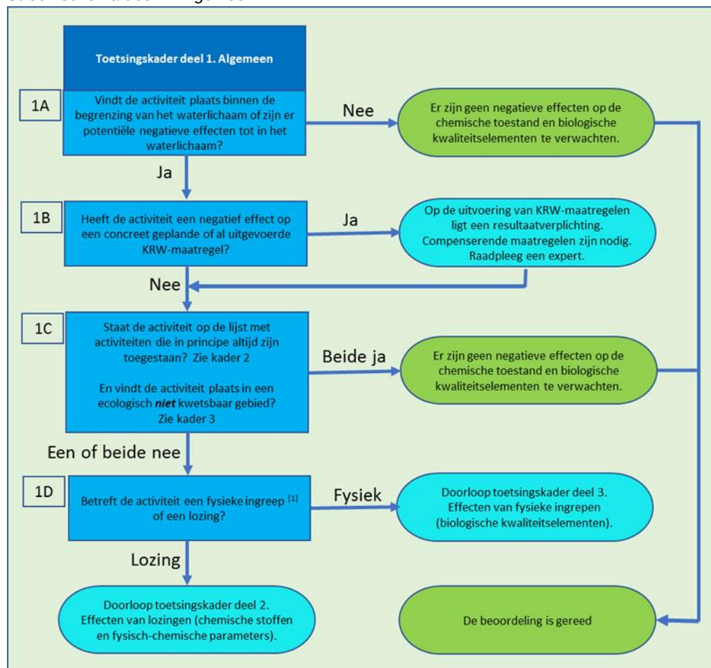
Stroomschema deel 1: Algemeen
