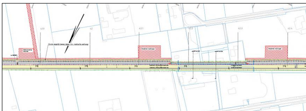
Figuur 9 Bouwweg vanaf de Frieslandweg naar werkterrein km 41.87 (let op noordpijl voor juiste oriëntatie).
