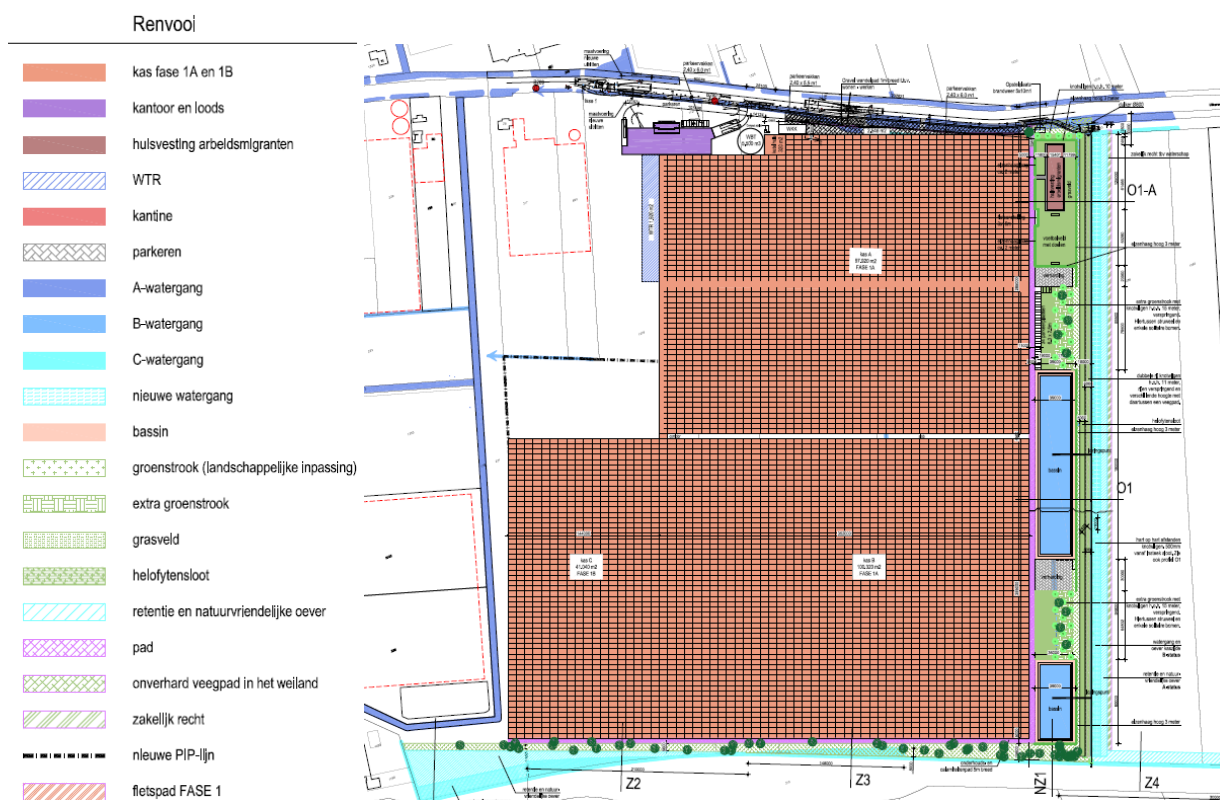
Afbeelding: Inrichtingstekening toekomstige situatie; (Bron: Ermstrang Bouwkundig ingenieursburo,)
