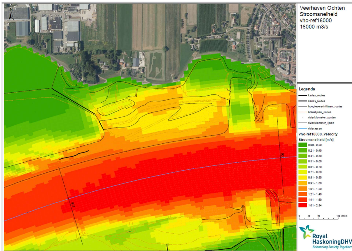
Figuur 6: Stroomsnelheid referentie bij 16.000 m³/s Lobith
