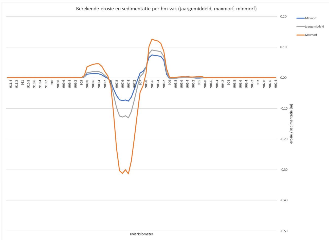
Figuur 15: Berekende erosie en sedimentatie per hectometer-vak (jaargemiddeld, maxmorf, minmorf) ten opzichte van de huidige situatie
