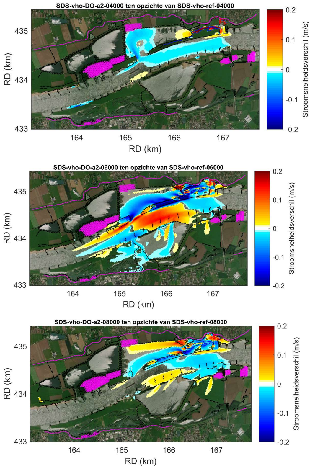
Figuur 14: Stroomsnelheidsverschil DO ten opzichte van referentie voor 4000, 6000 en 8000 m³/s bij Lobith
