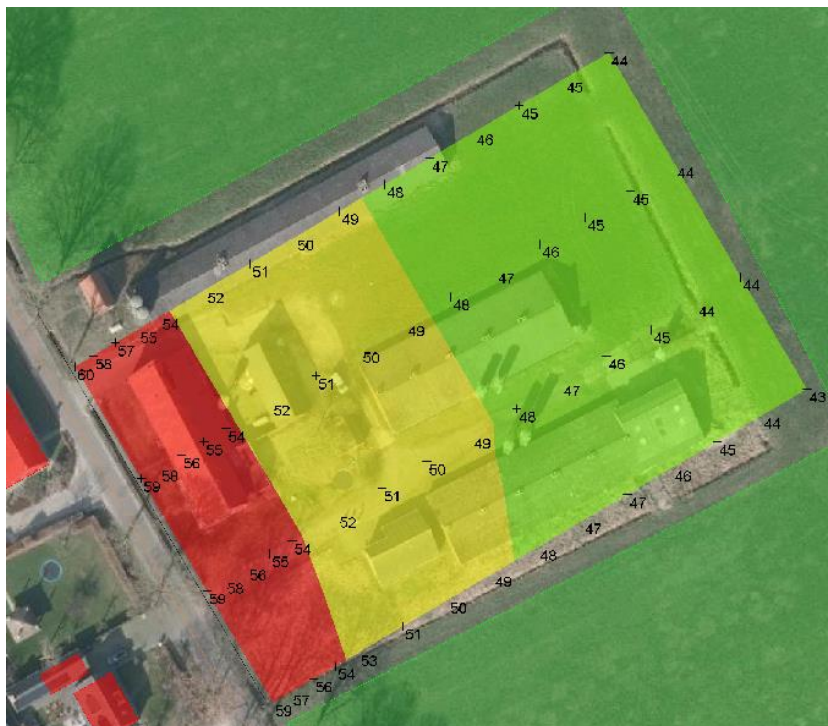
Figuur 4.3: Berekeningsresultaten Broekstraat op 7,5 meter (in dB).
