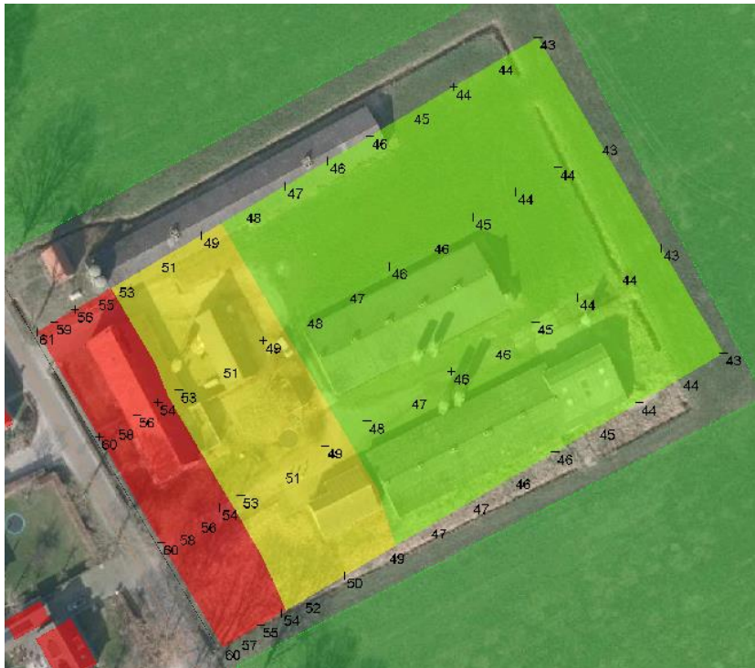
Figuur 4.2: Berekeningsresultaten Broekstraat op 4,5 meter (in dB).
