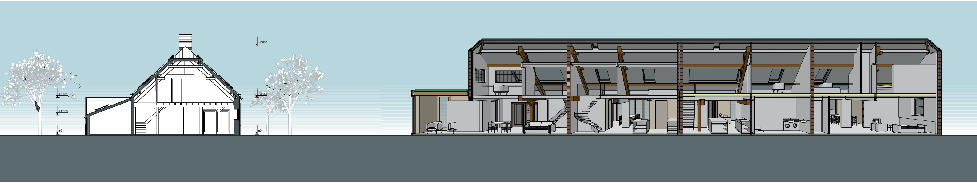
Dwarsdoorsnede AA bestand
